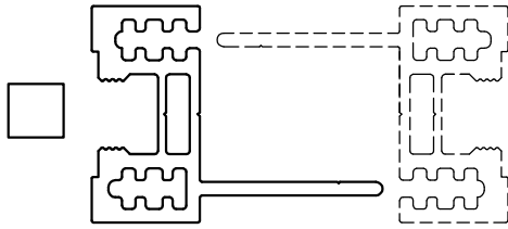
Trennwandprofil "simpel & clever"
